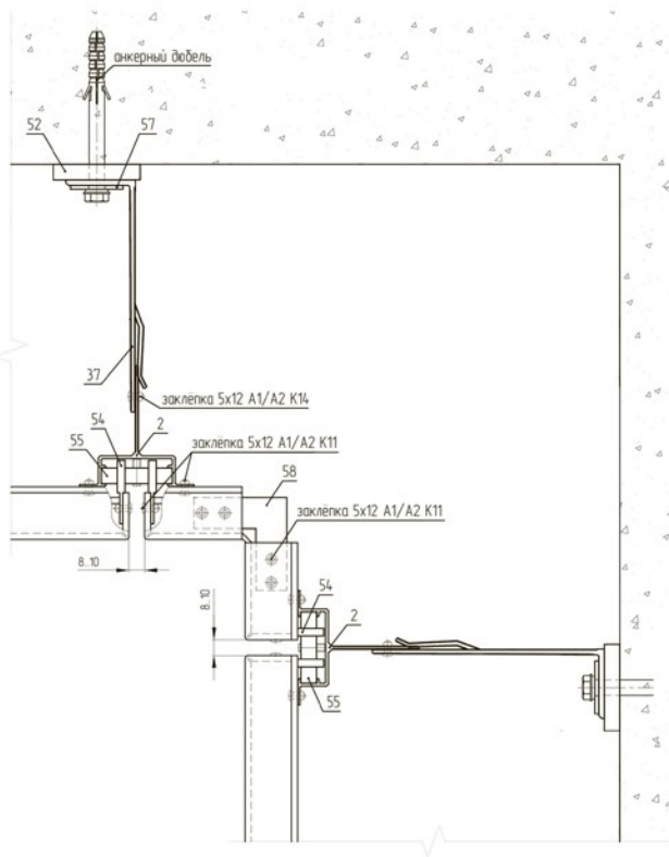
Узел облицовки внутреннего угла
