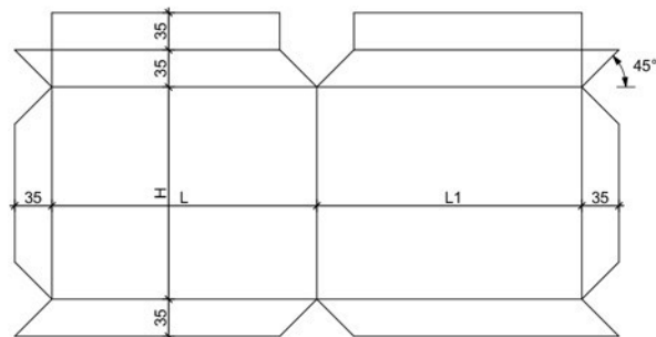
Угловая фасадная кассета
