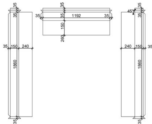
Откосы двери
