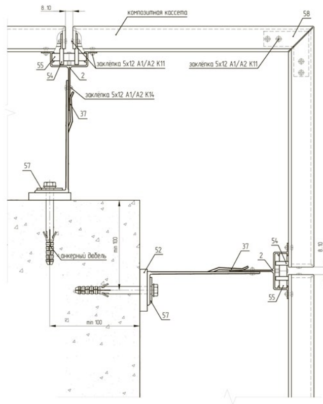
Узел облицовки наружного угла
